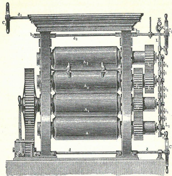
Fig. 23. Kalander mit vier Walzen.
