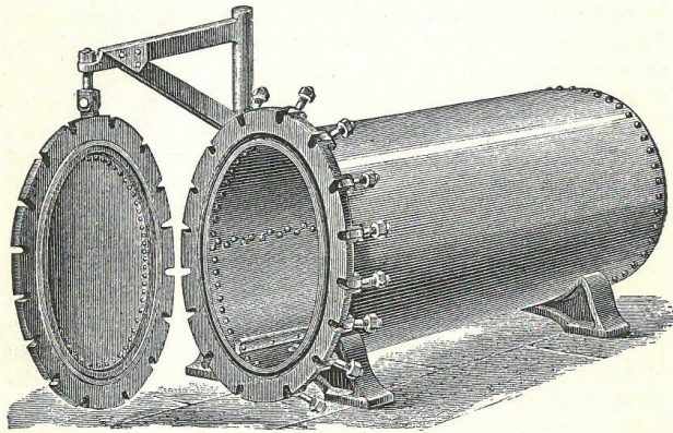
Fig. 25. Vulkanisierkessel.
